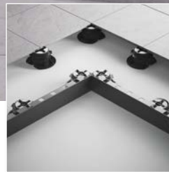
Detail Verlegung Abschlussprofil Innenecke mit Prime®
