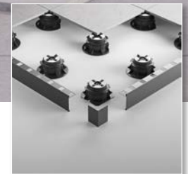
Detail Verlegung Abschlussprofil Außenecke mit Prime®
