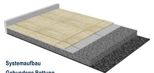
Systemaufbau Ungebundene Bettung
