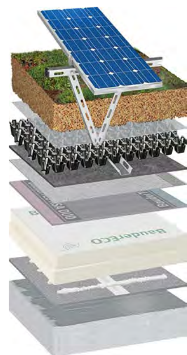
Bauder Flachdachaufbau mit BauderSOLAR G LIGHT
