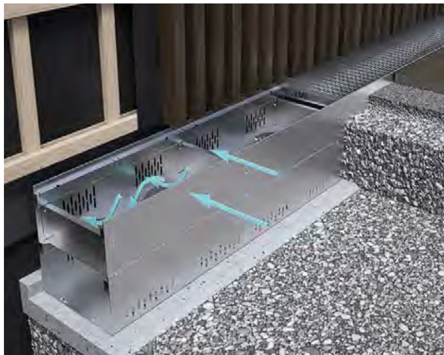
Sockelrinne sorgt für die Belüftung der Fassade
